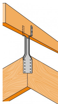
Fixation au droit de la charpente
