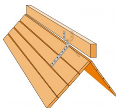
Fixation suivant pente de la toiture (pliable sur chantier)
